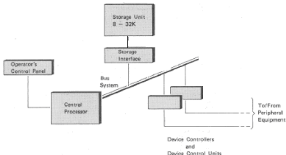
Typisk busskonfiguration
