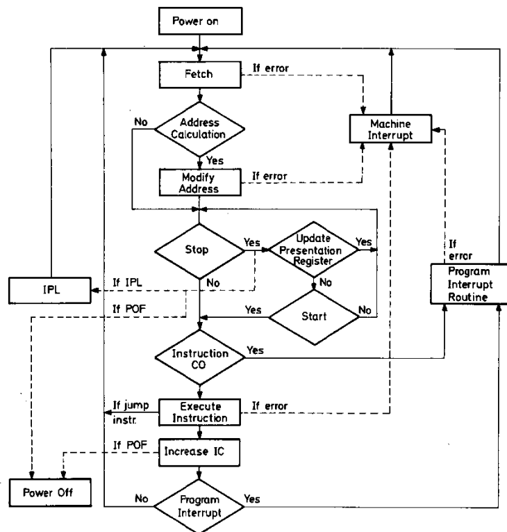
Styrenhetens flödesschema
